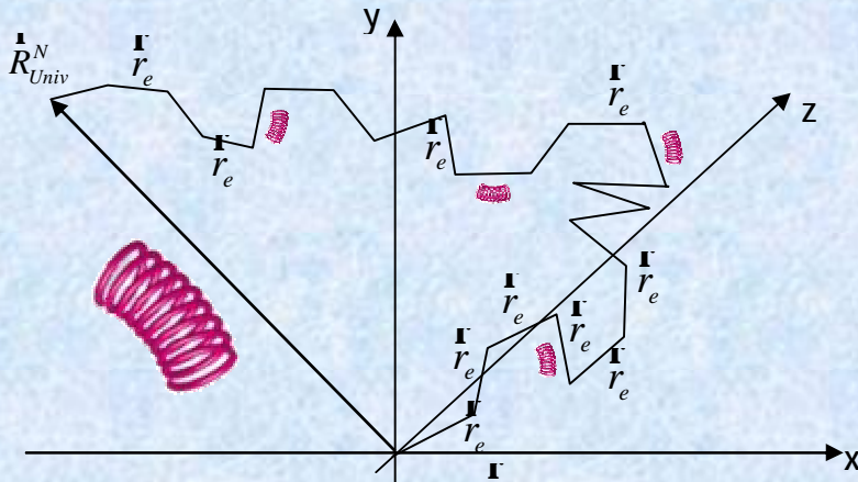
Fig. 5.2: Composizione delle N micro oscillazioni \mathbf{r}_e distribuite casualmente a formare l'oscillazione globale R_{Univ} .
