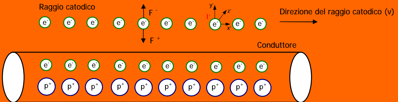
Fig. 1.3: Conduttore non percorso da corrente, visto dal sistema di riferimento \dot{I} ( x', y', z' ) di quiete del raggio catodico.
